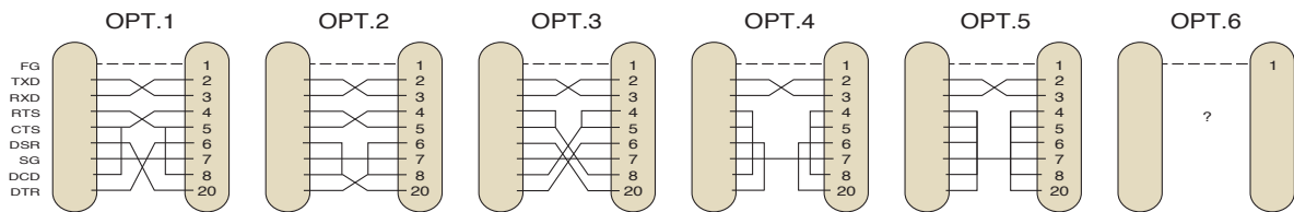
OPT.6 All the wiring except for Pin No. 1 can be designated at your free choice. 1以外の結線はすべてご自由に指定できます。専用の注文用紙をご利用ください。
